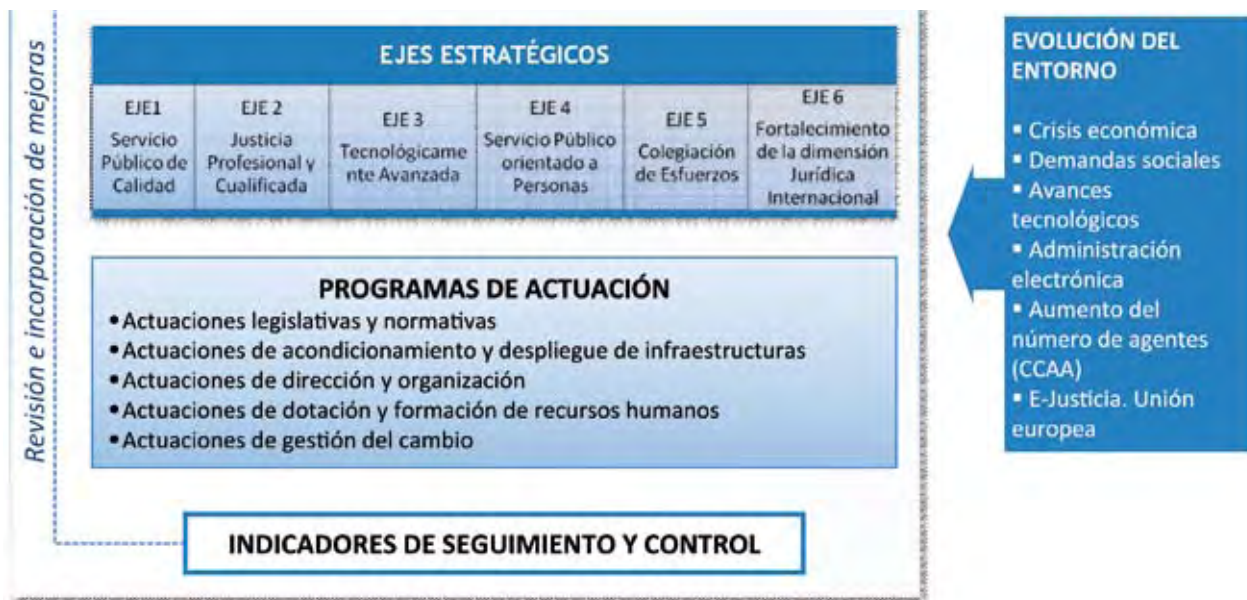
FIGURA 1. Esquema metodológico
