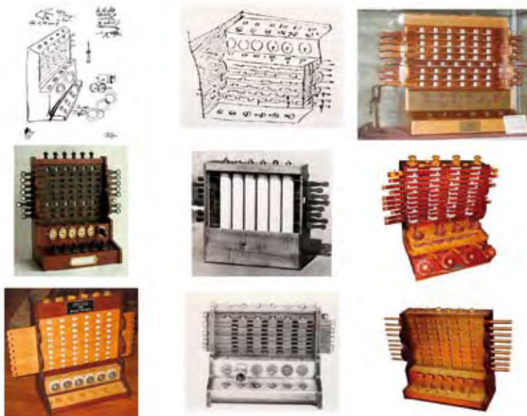
FIGURA 3. Bocetos originales y réplicas actuales de la máquina de Schickard
